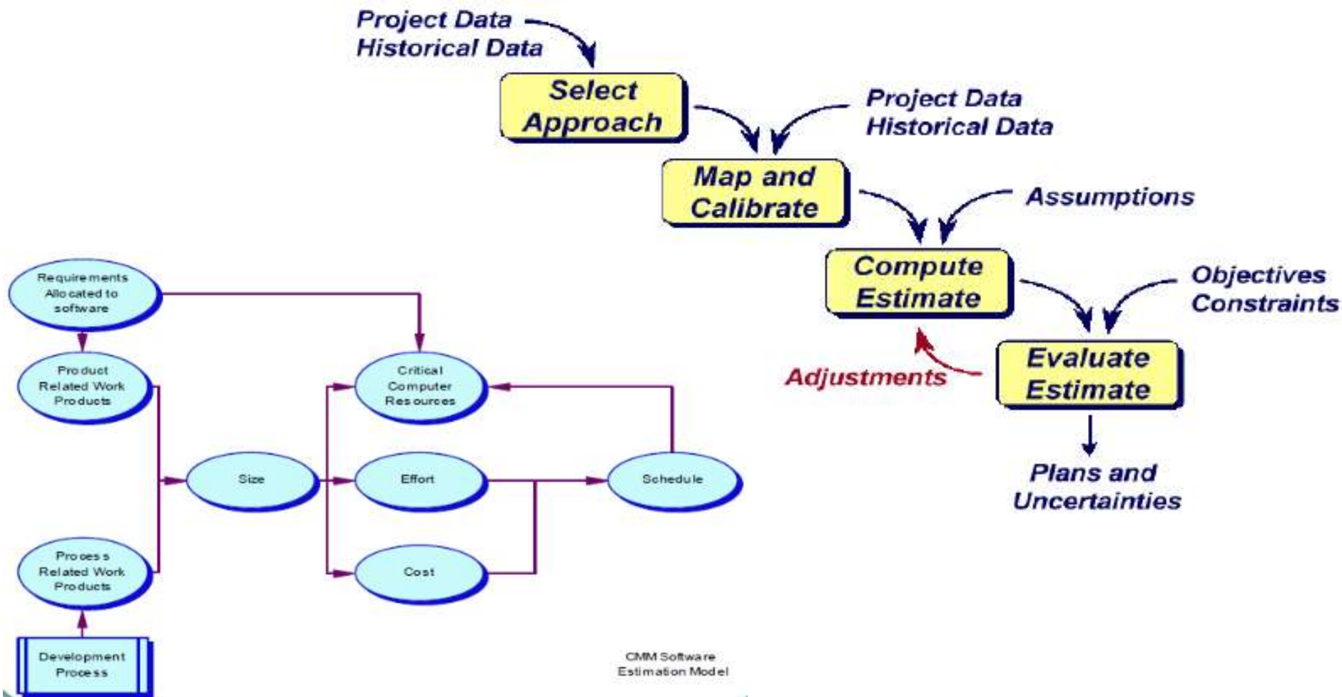
CMM软件估算模型
